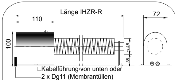
IHZR-R ohne Abdeckung
