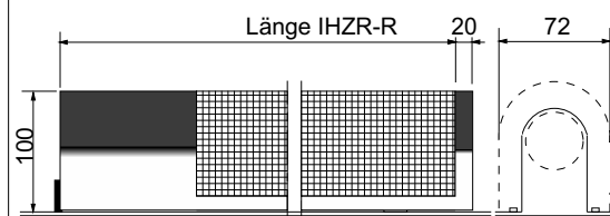
IHZR-R mit Abdeckung
